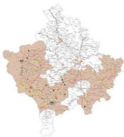
► Fig.4. - Lokalitetet arkeologjike - Shtrirja hapësinore
