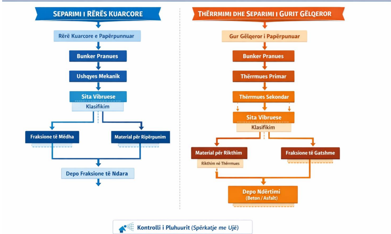
Fig. 6. Skemat e procesit teknologjik të seperacionit dhe therrmimit dhe klasifikimit
