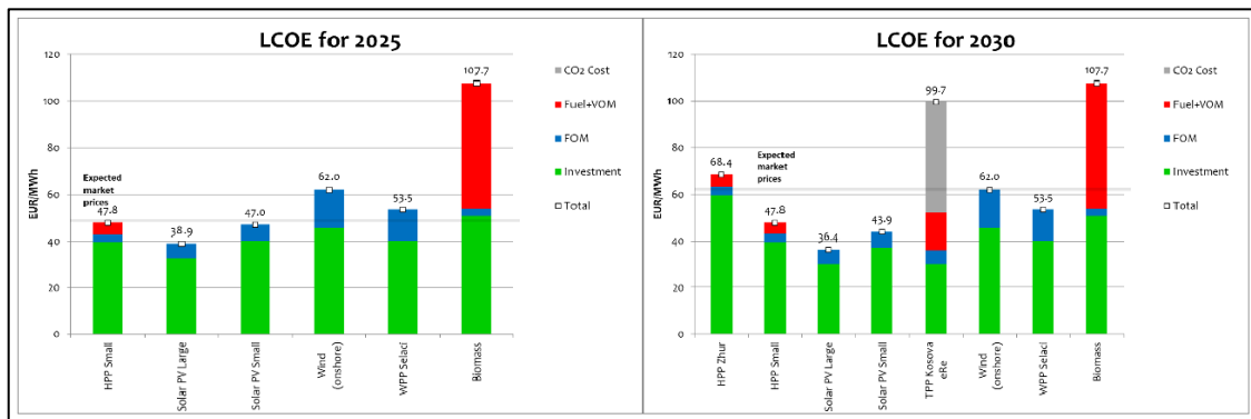
Figura 17. LCOE e vlerësuar e Opsioneve të Prodhimit të Energjisë në 2025 dhe 2030.
