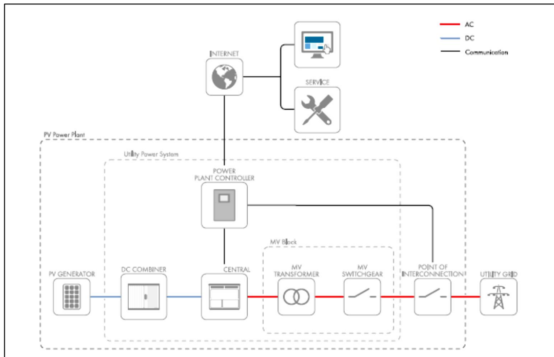
Figura 12.Diagrama Skematike e Impiantit.
