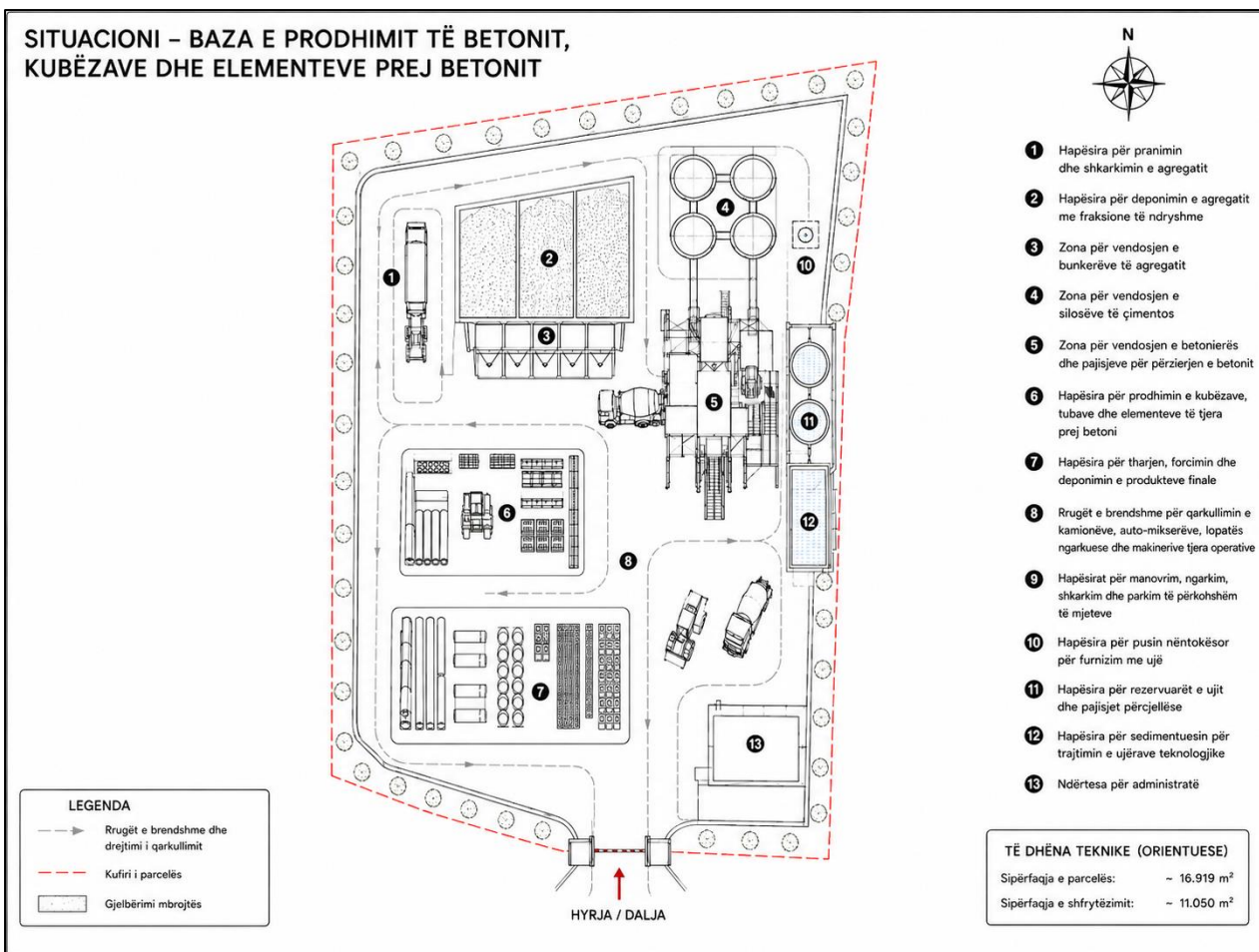
Figura 7. Plani i situacioni
