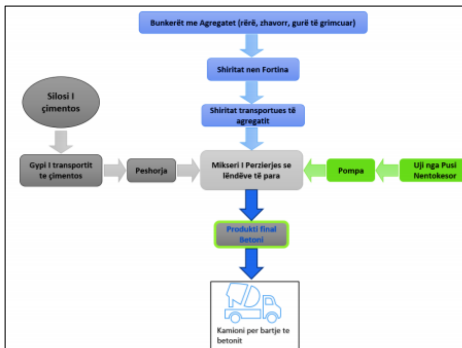
Figura 1. Procesi teknologjik i Punës së bazës për prodhimin e betonit
