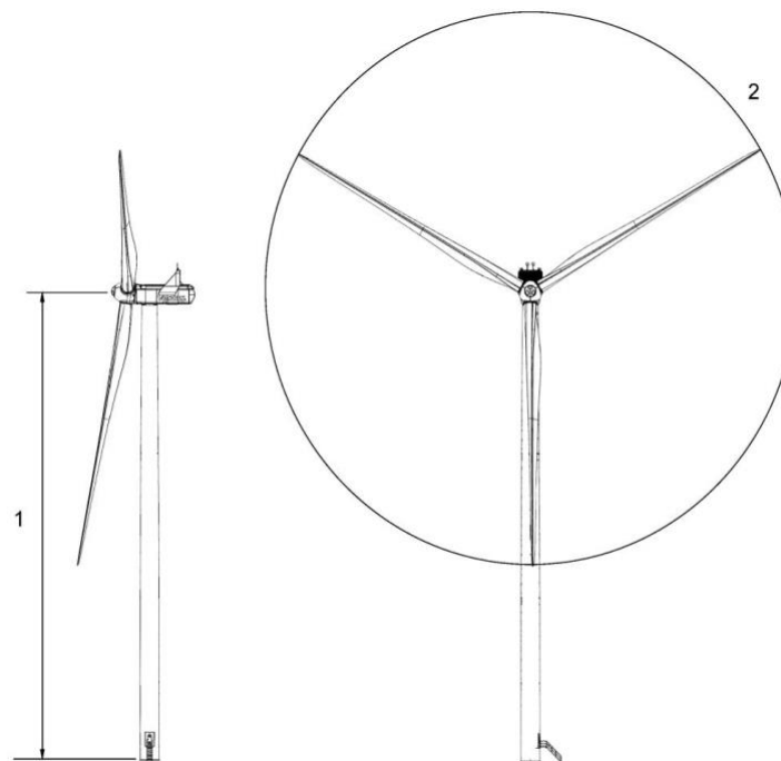
Fig 1. Dimensionet e turbinës GE 3.8-137
