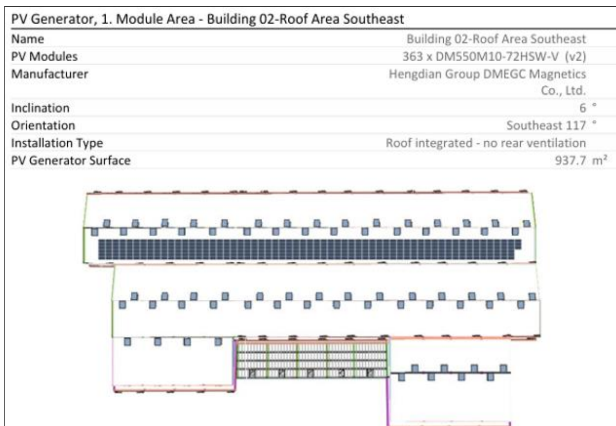
Figura 10 Orientimi i paneleve diellore fotovoltaike dhe kapaciteti i tyre
