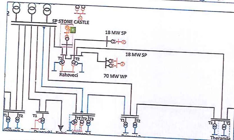
Figura 3. Skema njëpolare e kështjës së PS “STONE CASTLE” me kapacitet 20 MW dhe baterisë akumuluese 3MW/6MWh.
