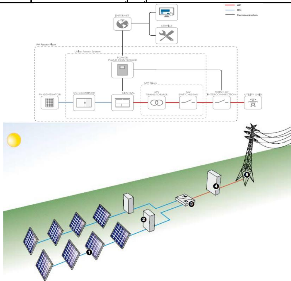
Skema e procesit të impiantit Solar 3.5MW
