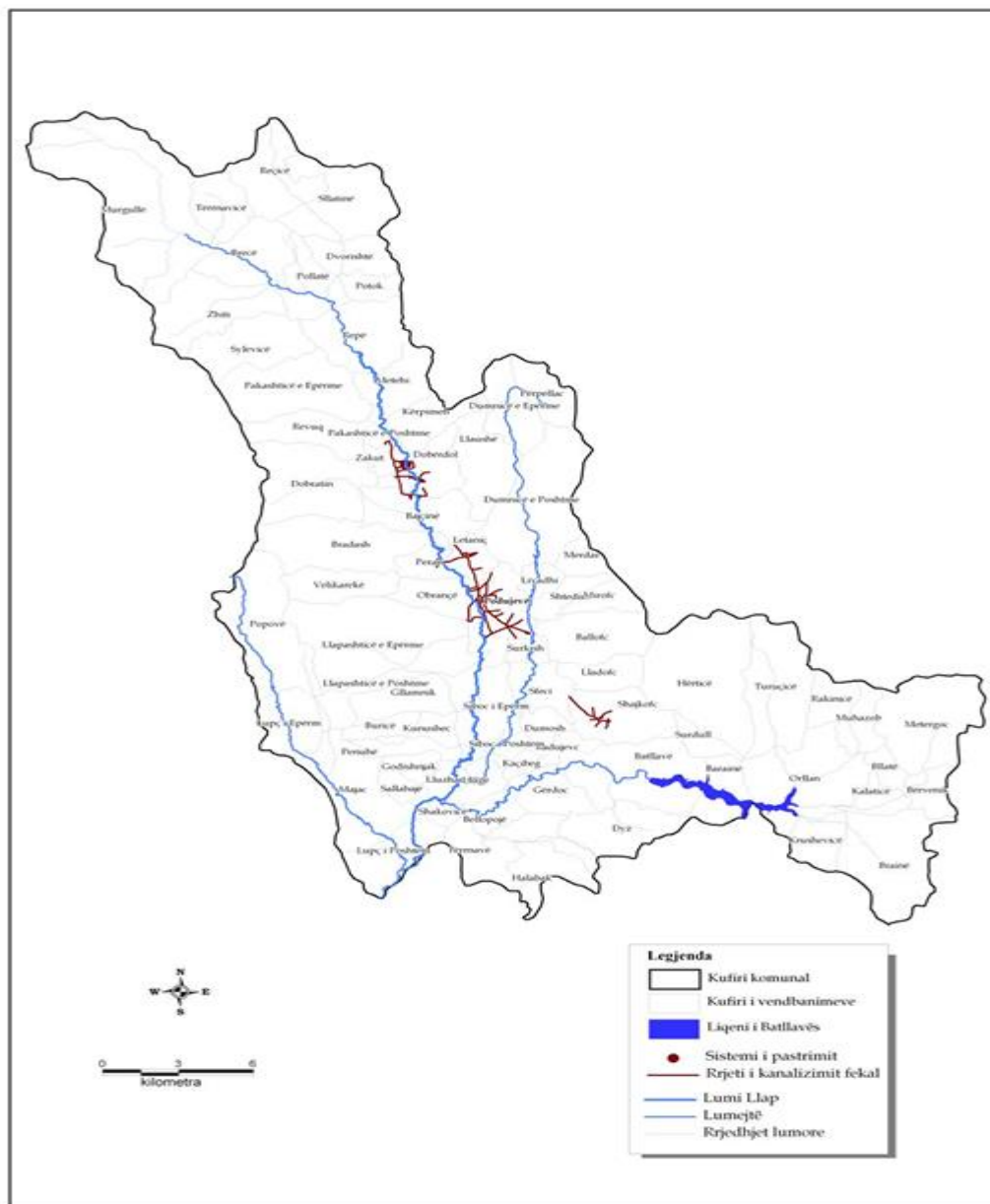
Figura 16. Rrjeti i kanalizimit
