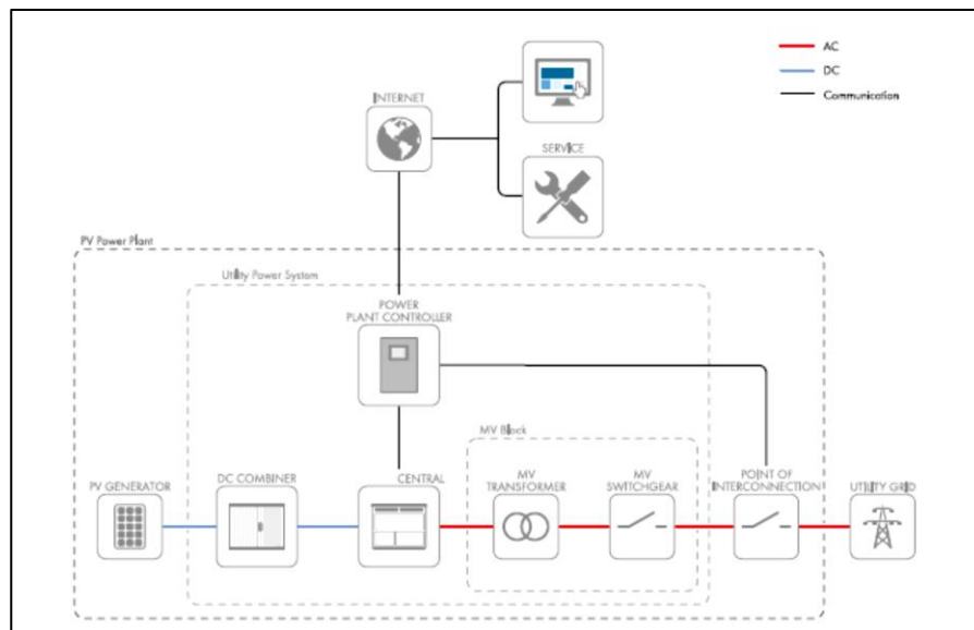
Figura 12. Diagrama Skematike e Impiantit
