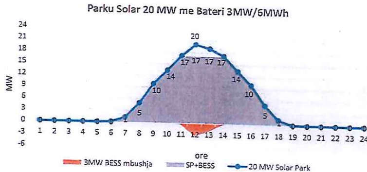
Figura 2. Ndikimi i Baterisë akumuluese 3MW(6MWh) në reduktimin e fuqisë dalëse të Parkut Solar nga 20 MW në 17 MW, gjatë prodhimit maksimal.
