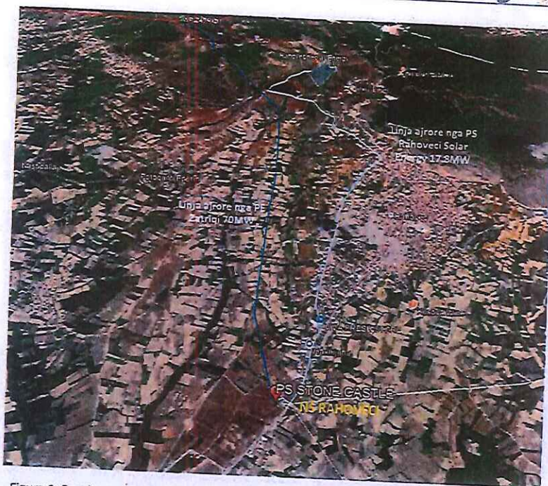
Figura 1. Pamja nga Google Earth e Parkut Solar “STONE CASTLE” me kapacitet 20 MW, në relacion me rrjetin më të afërt – linjat transmetuese dhe nënstationet
