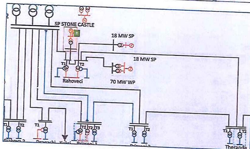
Figura 3. Skema njëpolare e kycjes së PS “STONE CASTLE” me kapacitet 20 MW dhe baterisë akumuluese 3MW/6MWh.
