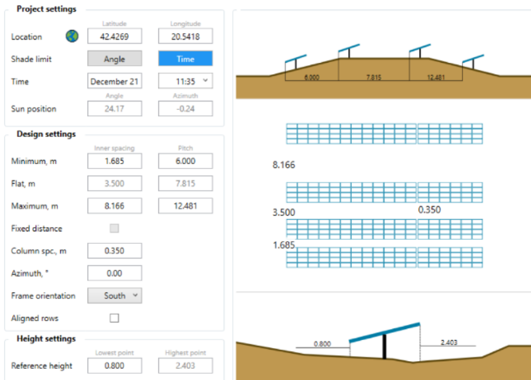
Struktura e ndërtimit për PV panelet
