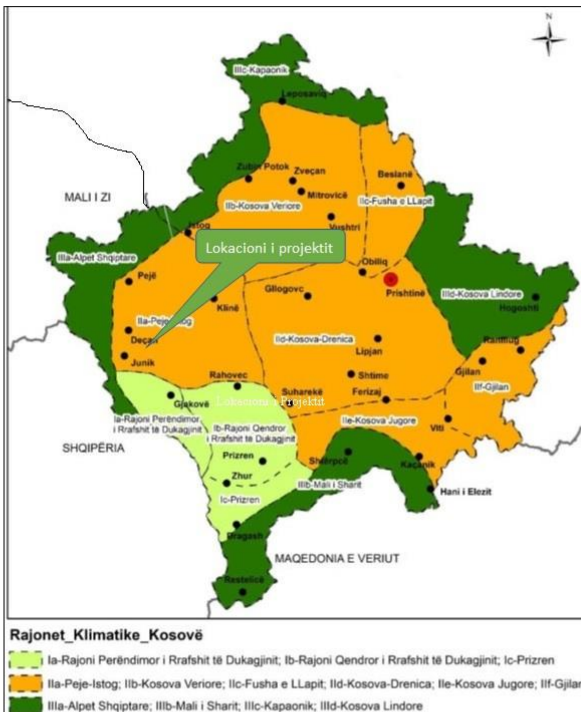
Figura 5: Rajonet Klimatike në Kosovë
