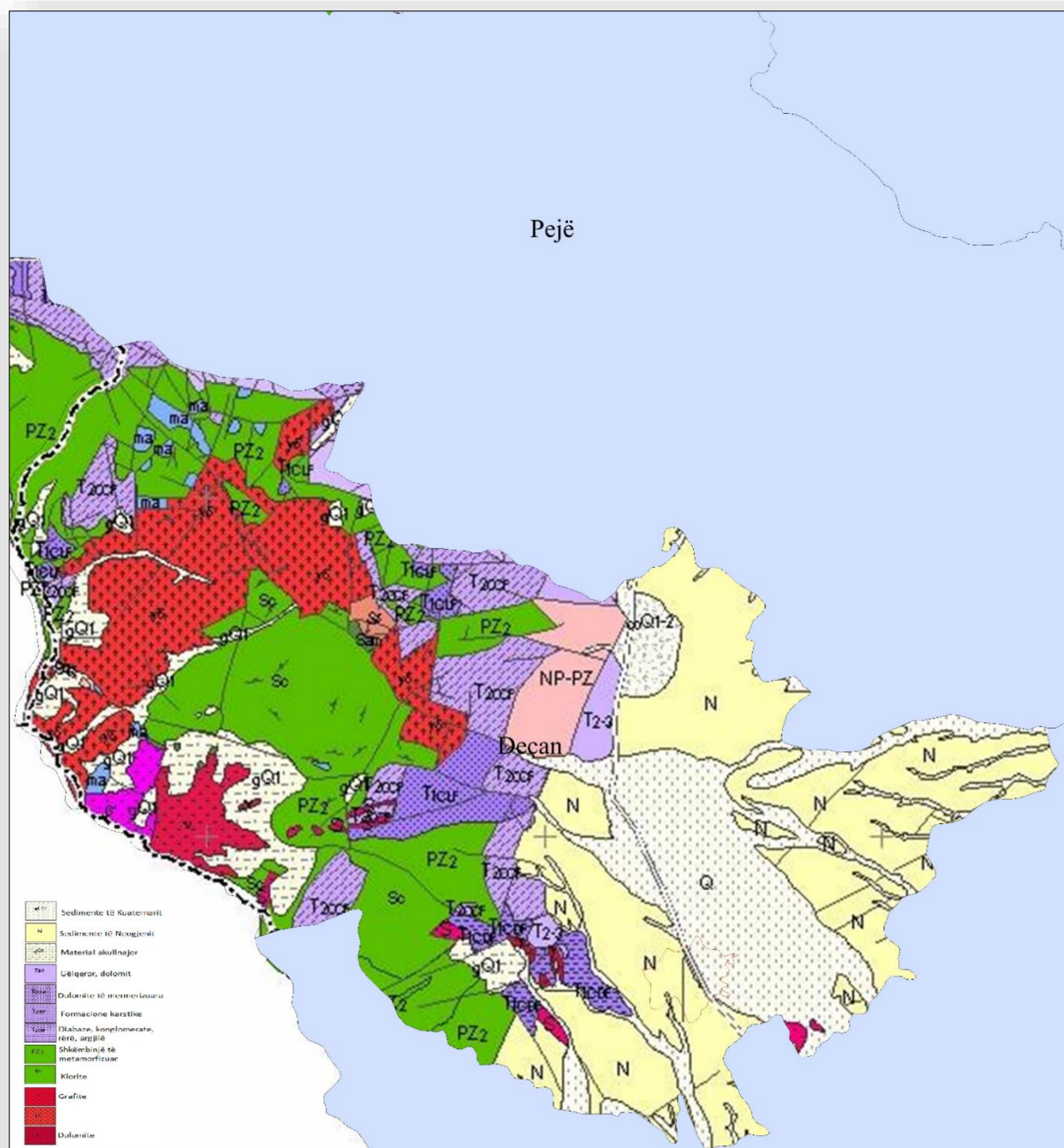
Figura 14: Harta gjeologjike e Deçanit
