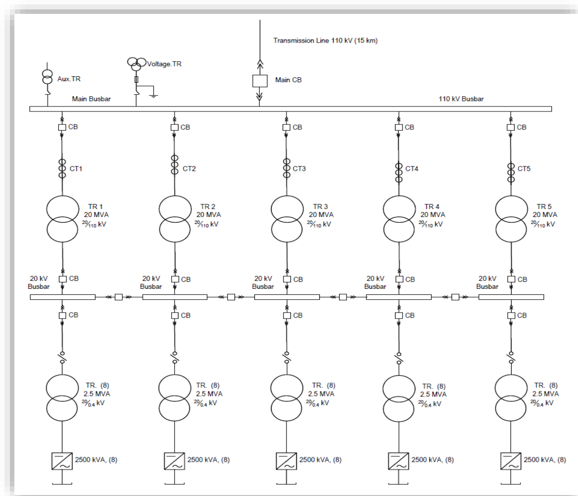
Figura 17: Skema Elektrike
