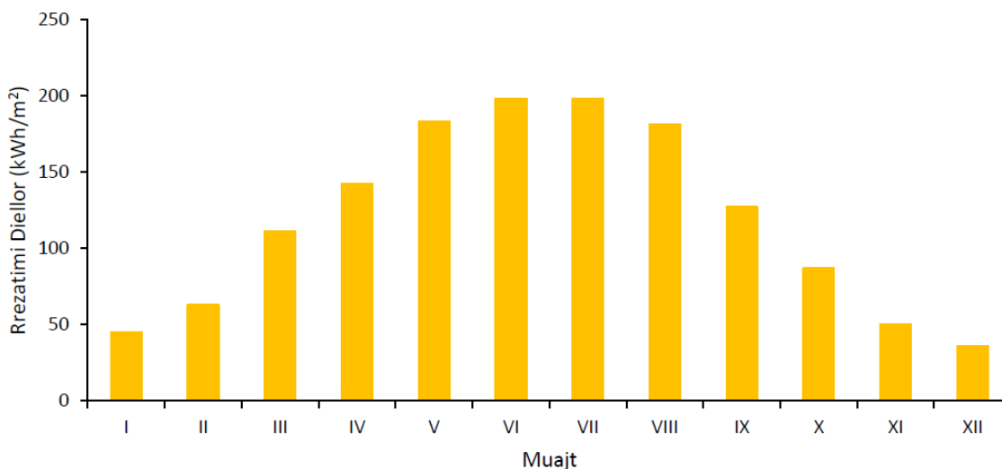
Figura 8: Shpërndarja Brenda vjetore e Rrezatimit Diellor, Meteonorm
