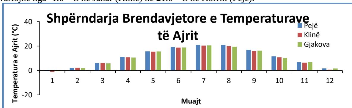
Figura 9: Shpërndarja Brenda vjetore e Temperaturave të Ajrit
