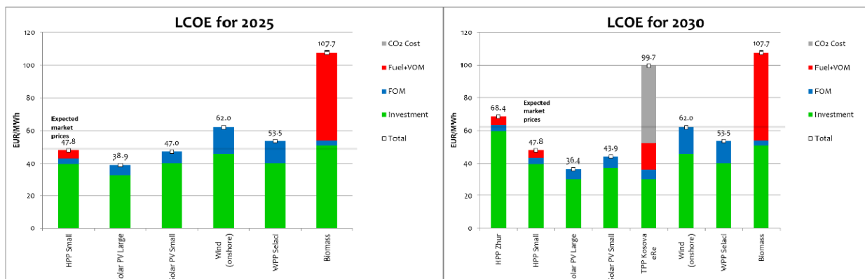
Figura 19: LCOE e vlerësuar e Opsioneve të Prodhimit të Energjisë në 2025 dhe 2030
